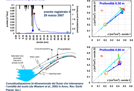
Distribuzione dell'umidità del suolo, a scala d'evento, lungo il transetto alle due differenti profondità
